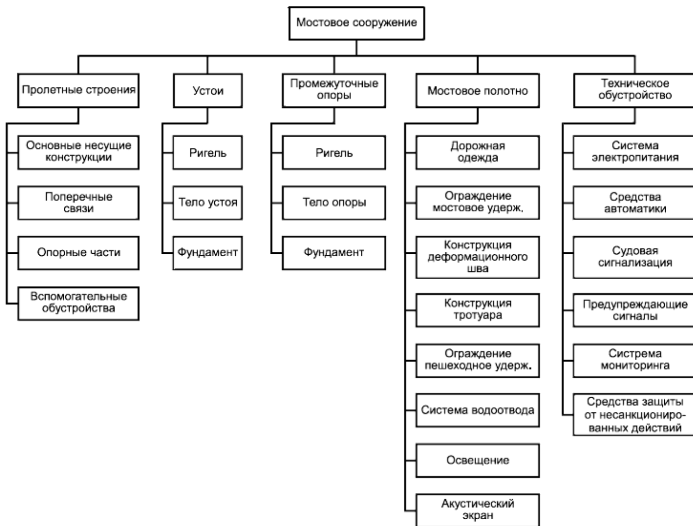
Рисунок А.1 - Структурная схема мостового сооружения
